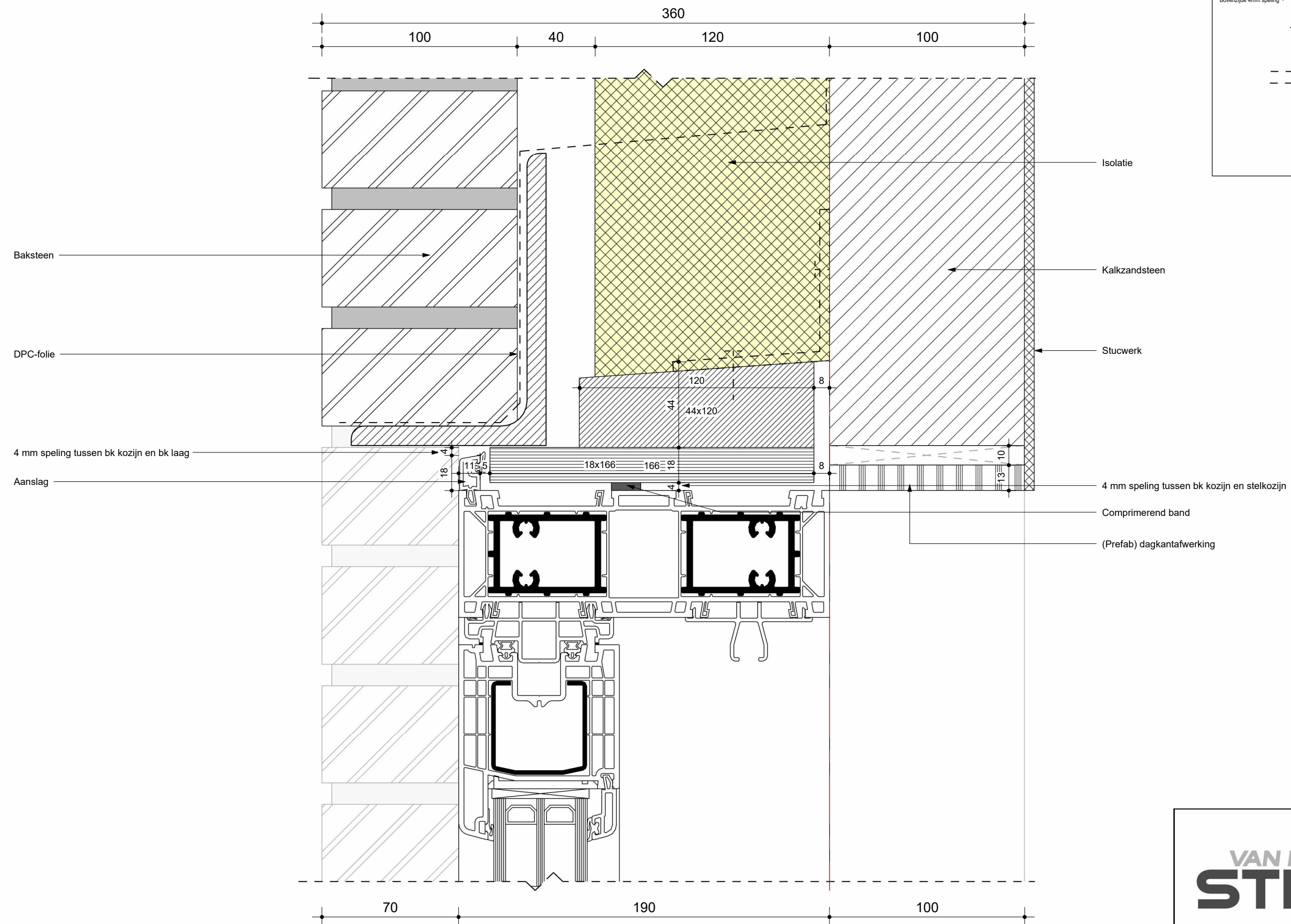
Inbouwdetail bovendorpel schuifdeur
